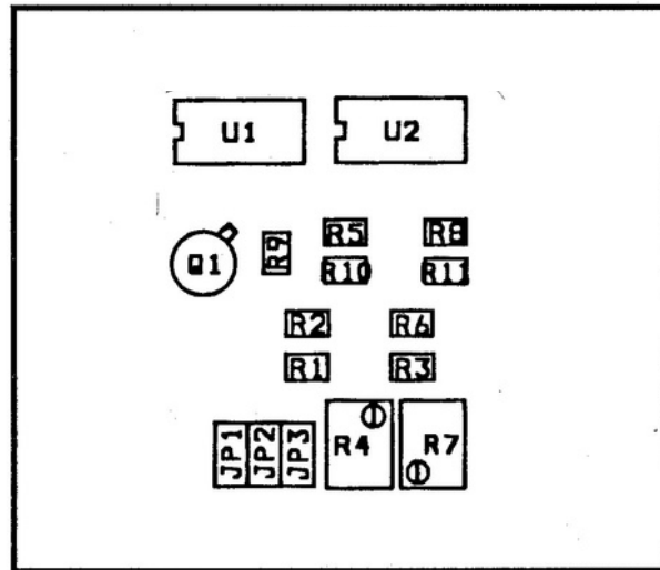
CL001 4-20mA Module Layout
